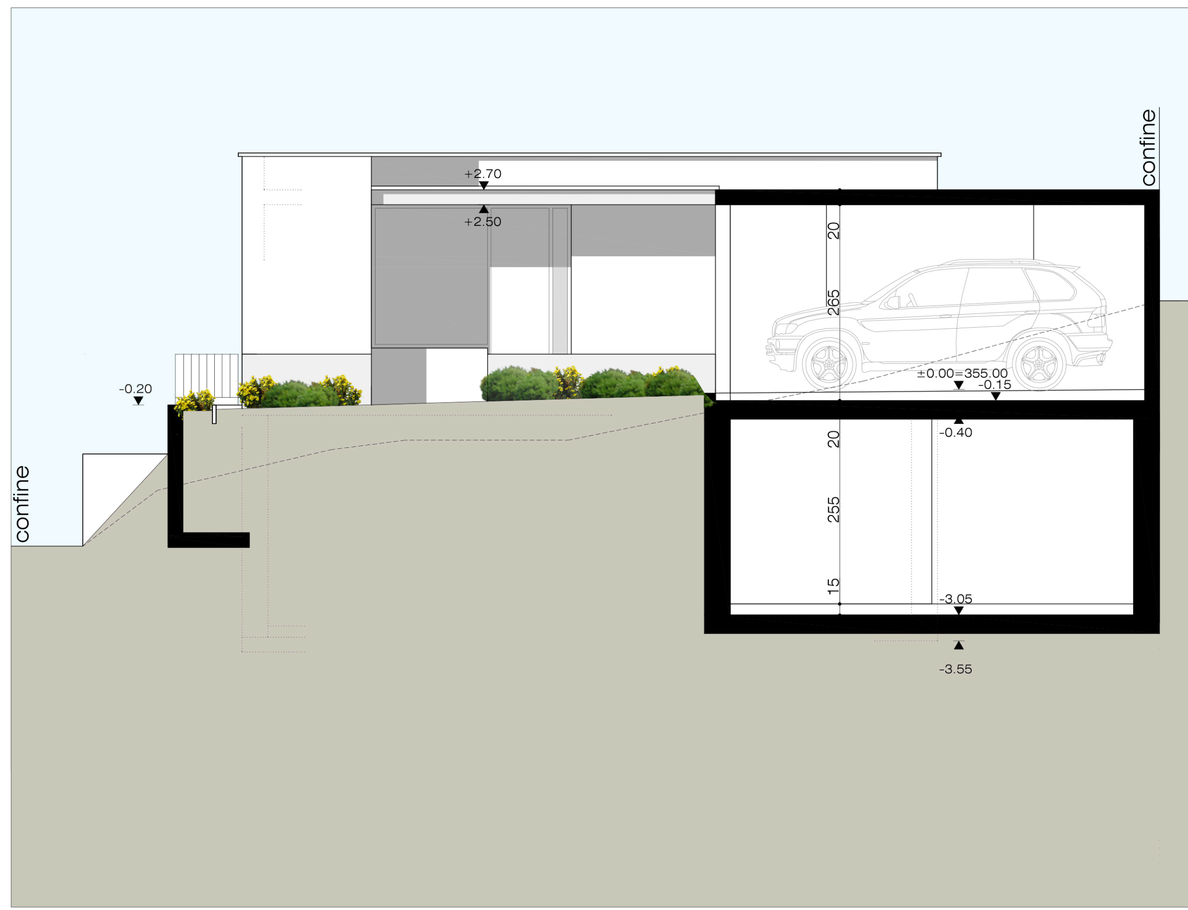
FACCIATA NORD
